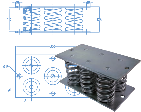
AISLANTES METÁLICOS / SPRING ISOLATOR ISOLANTS METALIQUES / FEDERISOLATOREN
